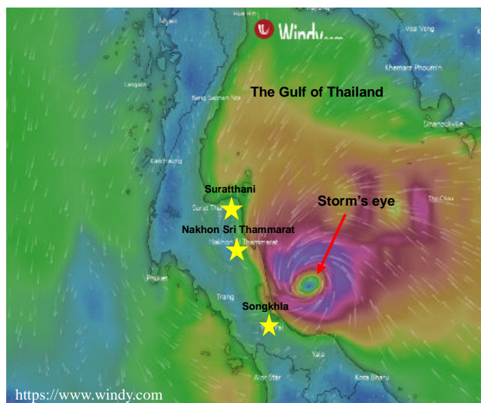
図 台風 Pabuk の位置 (2019 年 1 月 4 日 午前 9:00 現在)
